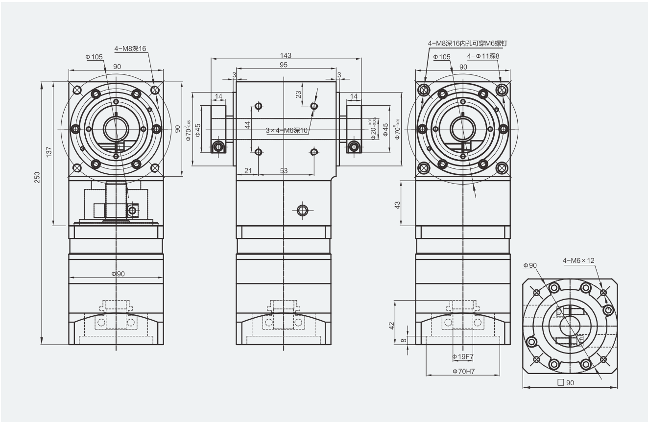
ZTB090-L2
