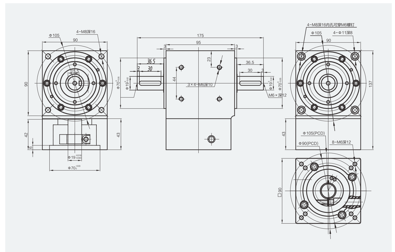
ZT090-L2
