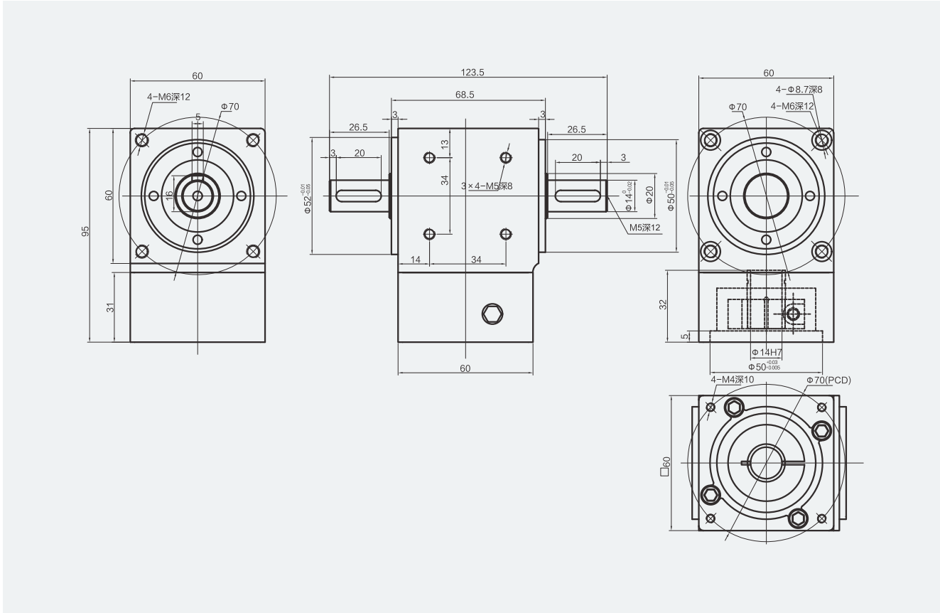
ZT060-L2
