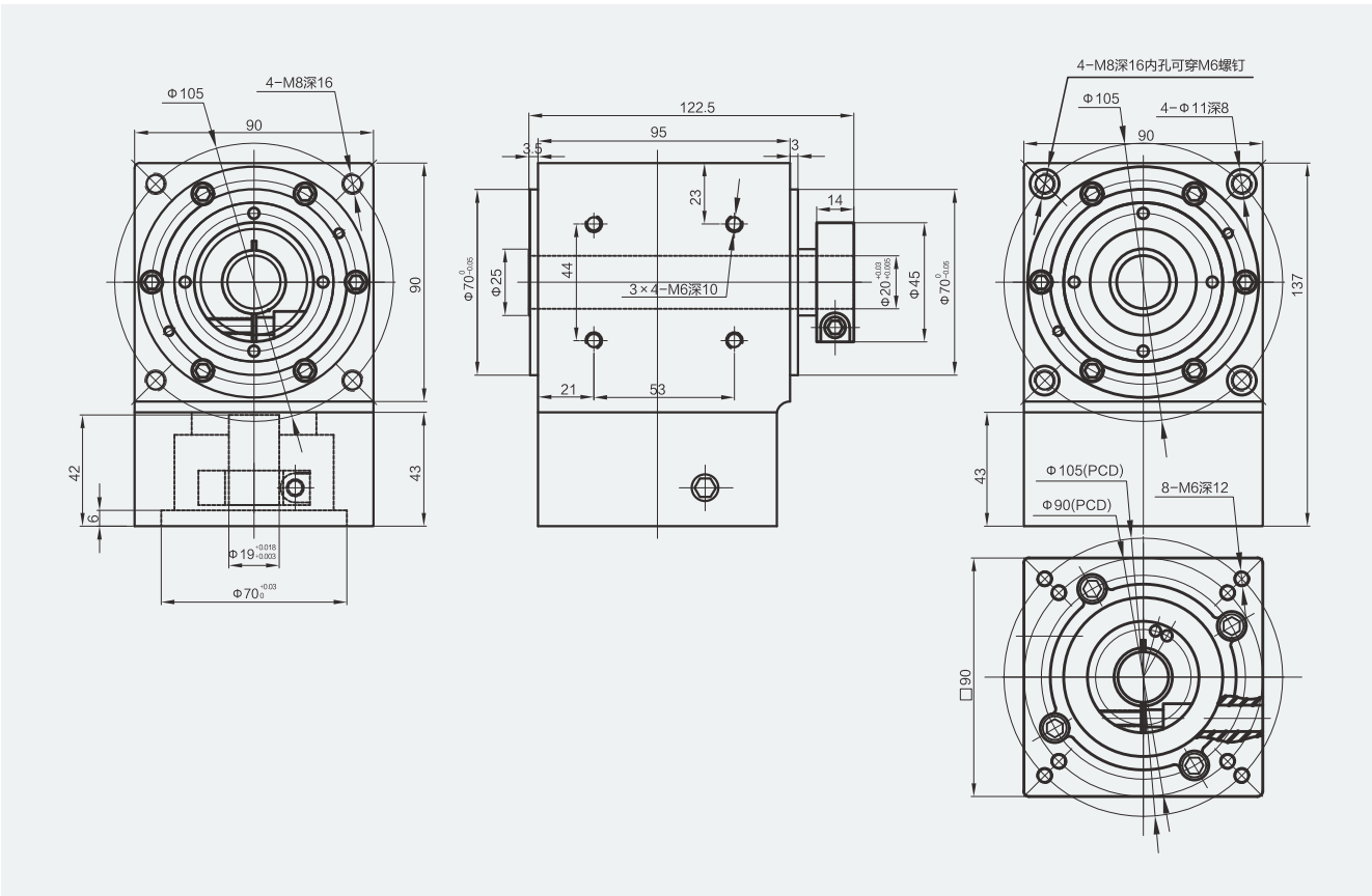
ZB090-L2
