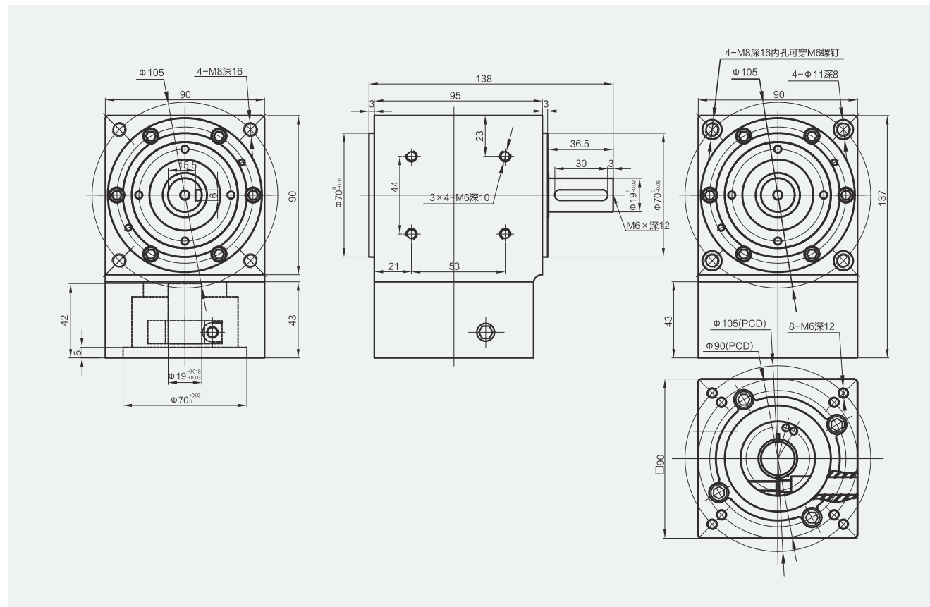
ZH090-L2
